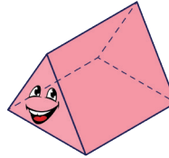
Üçgen Prizma
