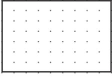
Dörtgen
