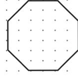
Sekizgen
