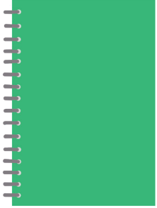
Dörtgen
