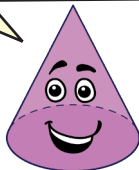
Koni
