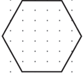
Altıgen
